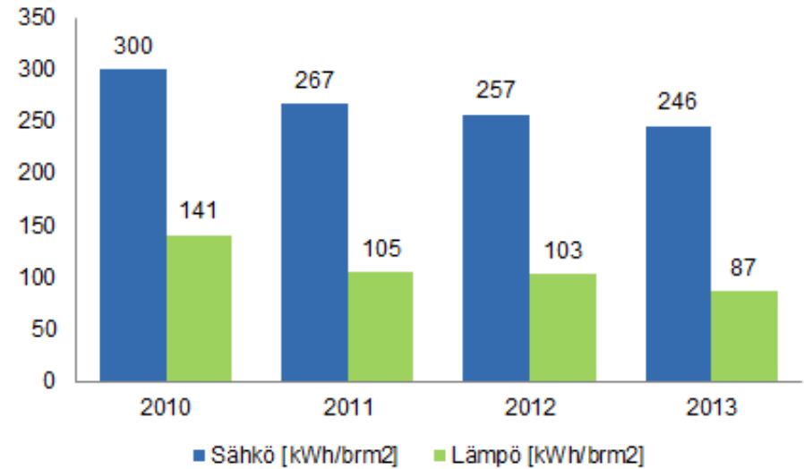
Sähkön- ja lämmönkulutus/brm2
